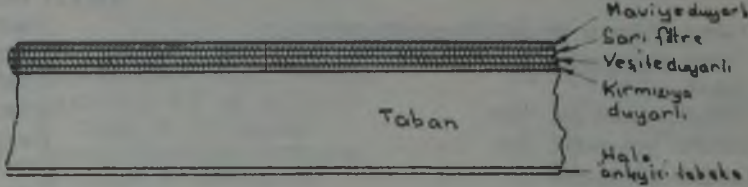
Şekil 5 : Monopak bir filmin kaba kesiti.
